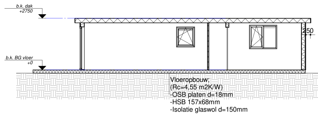
Doorsnede 1 1 : 100
