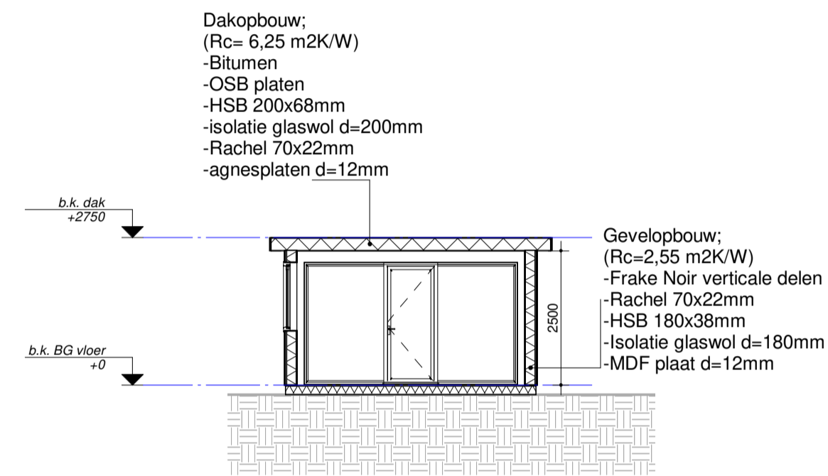
Doorsnede 2 1 : 100
