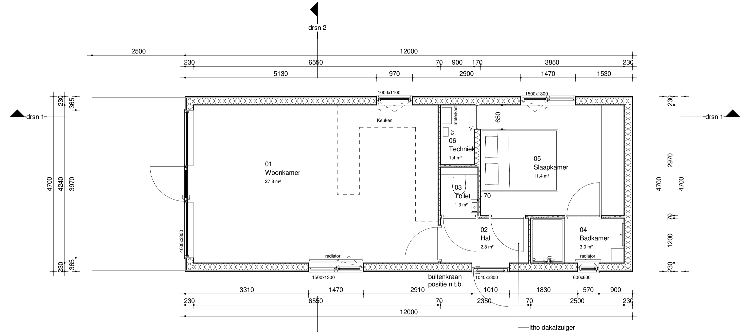
Begane grond vloer 1 : 50
