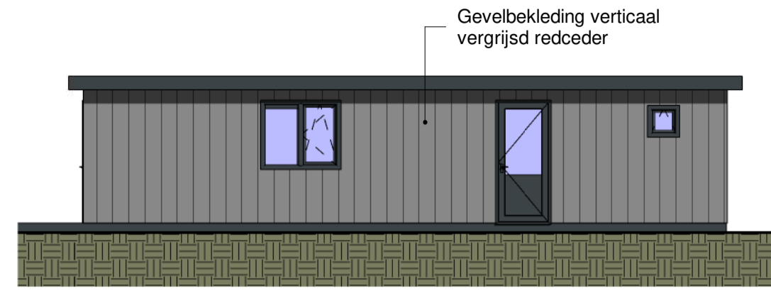
Voorgevel 1 : 100
