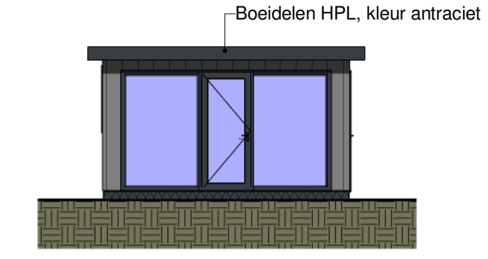
Linkergevel 1 : 100
