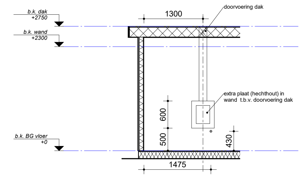
aanzicht gashaard 1 : 50
