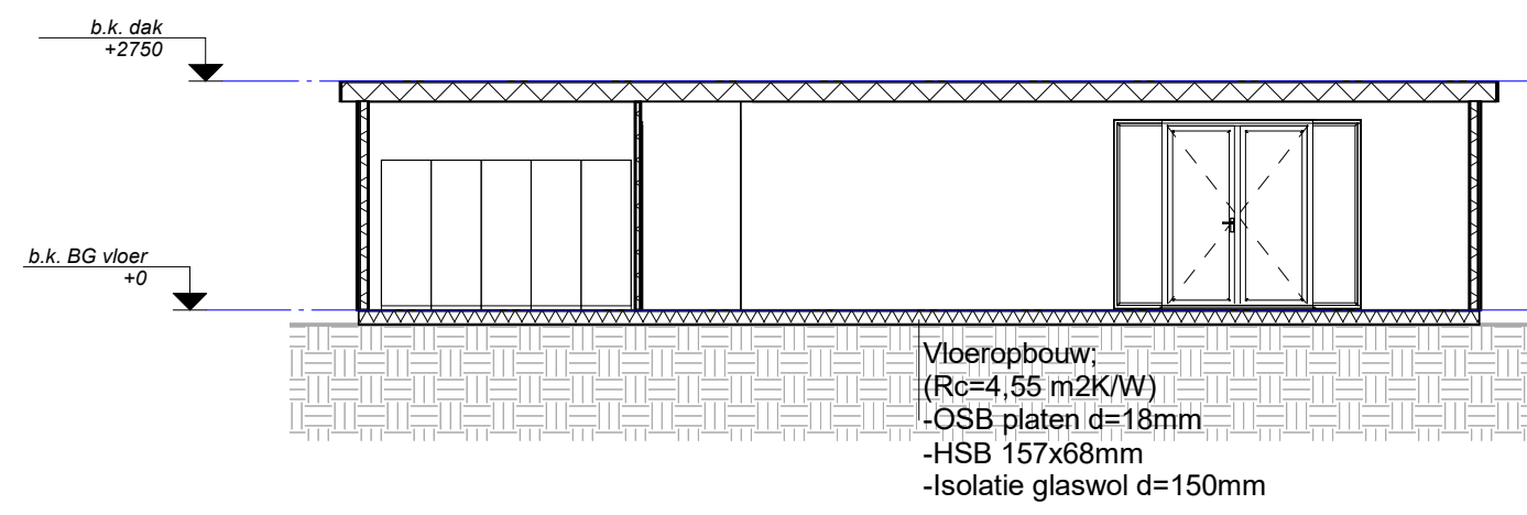
Doorsnede 1 1 : 100
