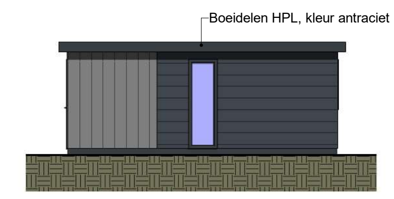
Linkergevel 1 : 100
