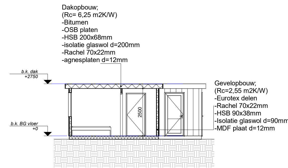
Doorsnede 2 1 : 100
