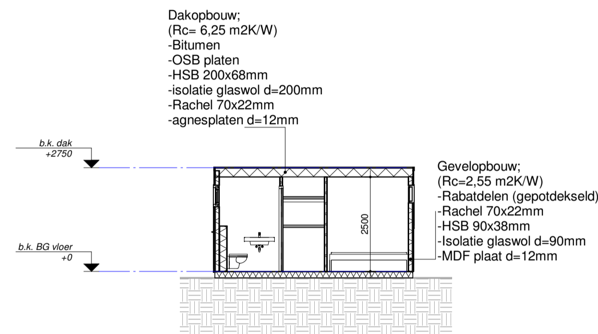
Doorsnede 2 1 : 100
