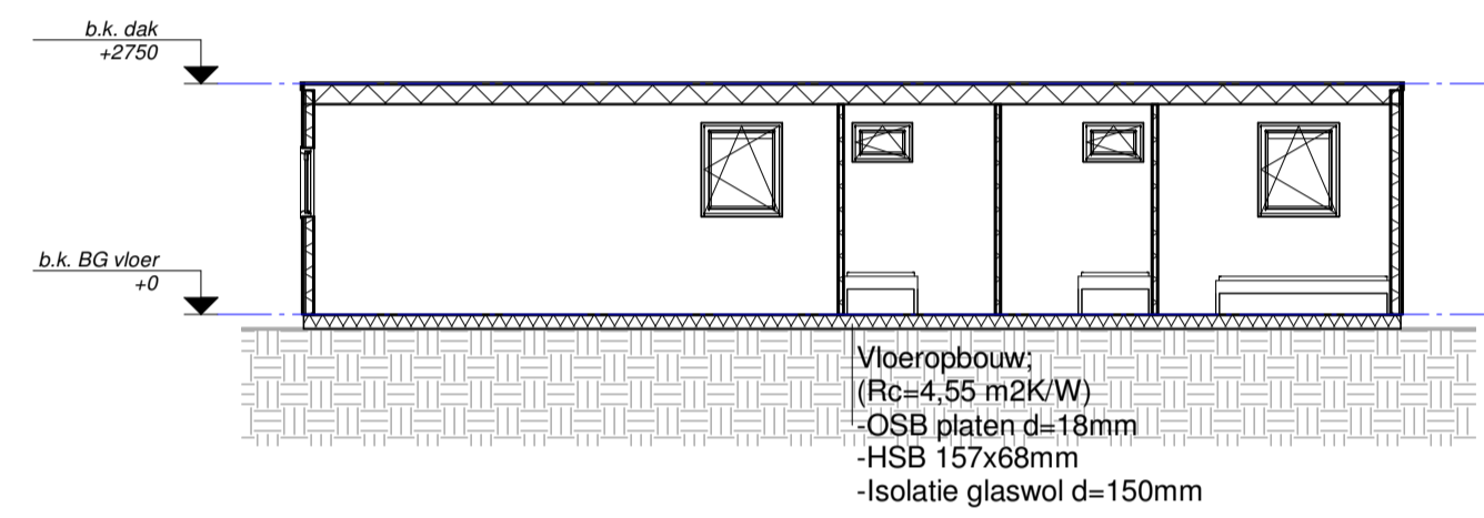
Doorsnede 1 1 : 100
