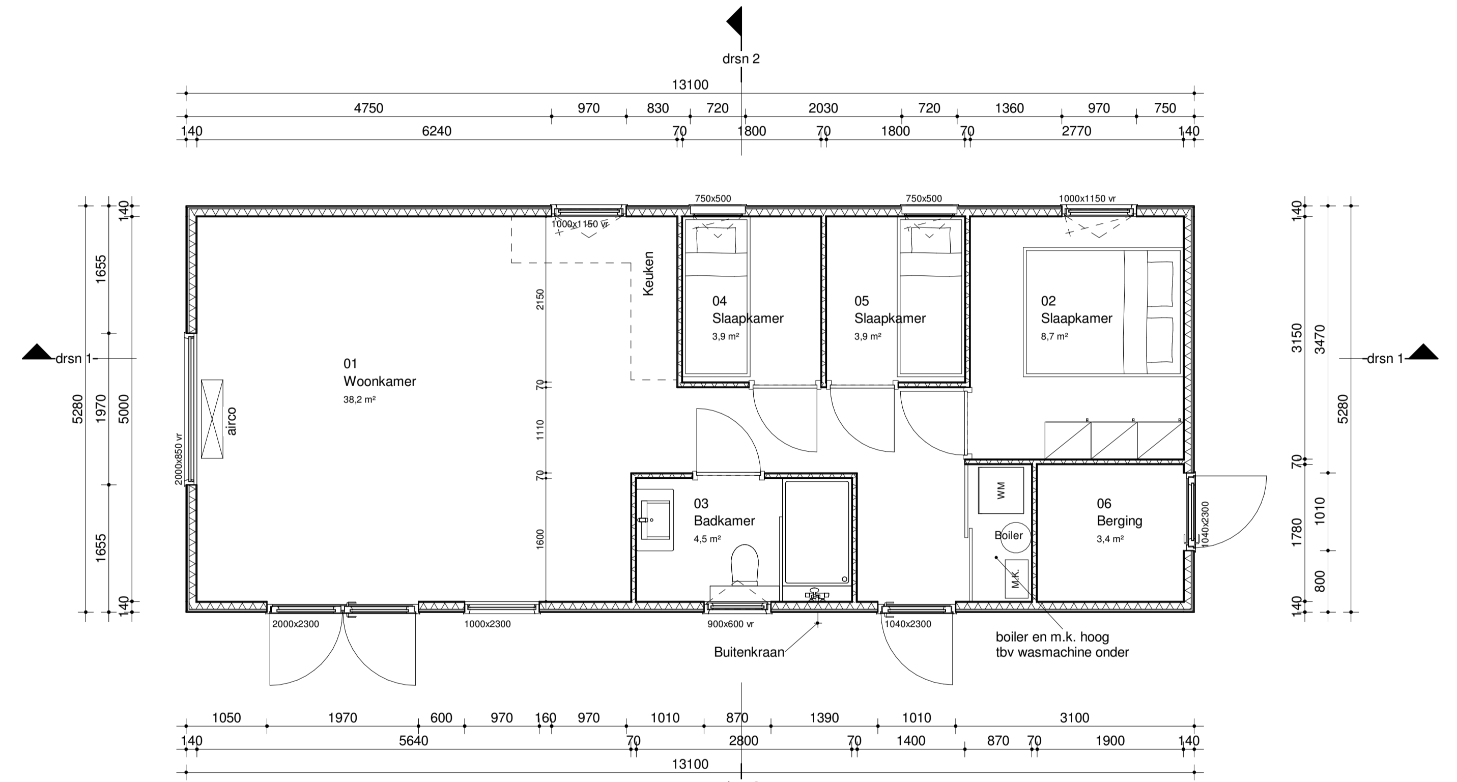
Begane grond vloer 1 : 50
