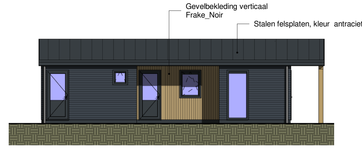
Achtergevel 1 : 100
