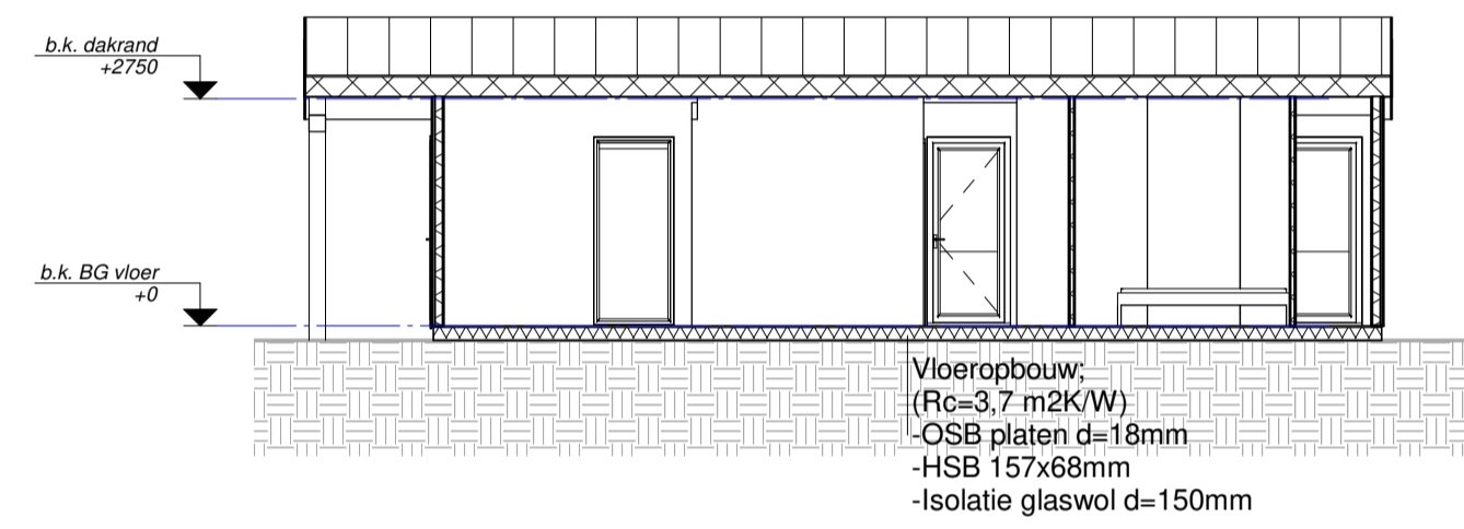
Doorsnede 1 1 : 100
