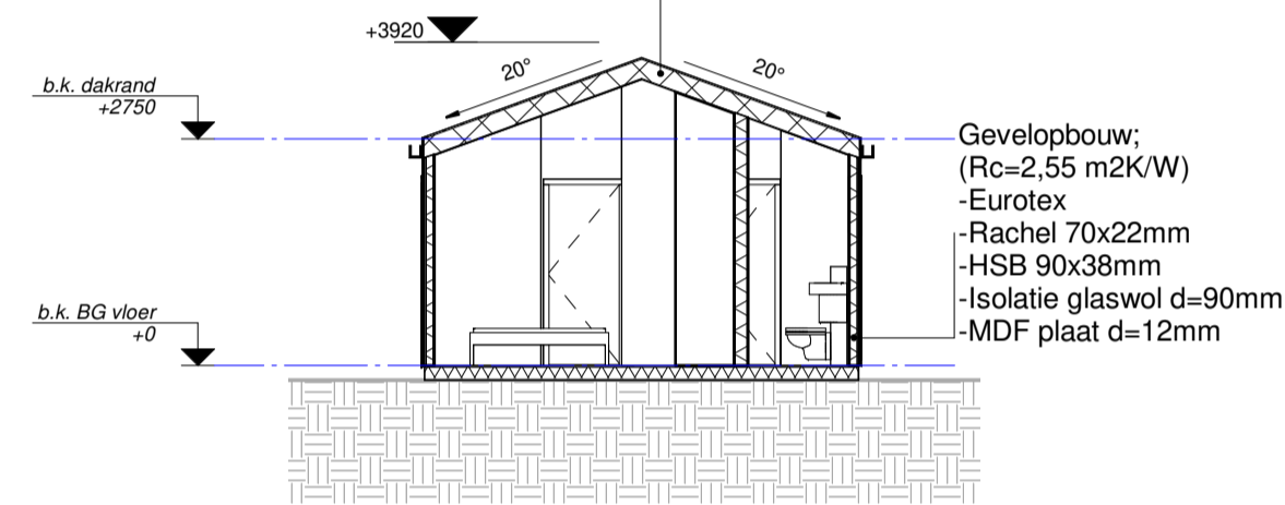
Doorsnede 2 1 : 100
