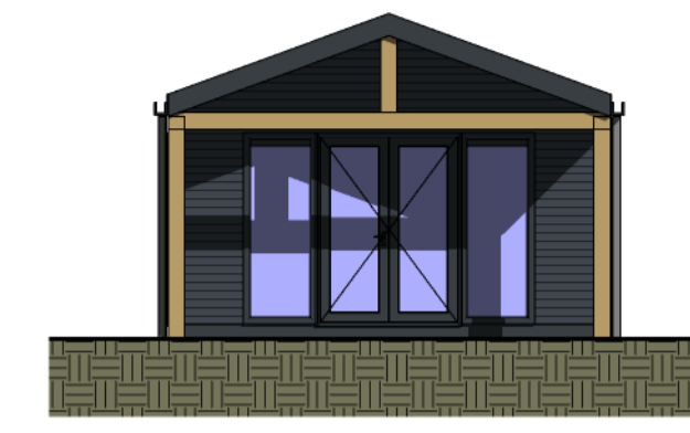
Linkergevel 1 : 100
